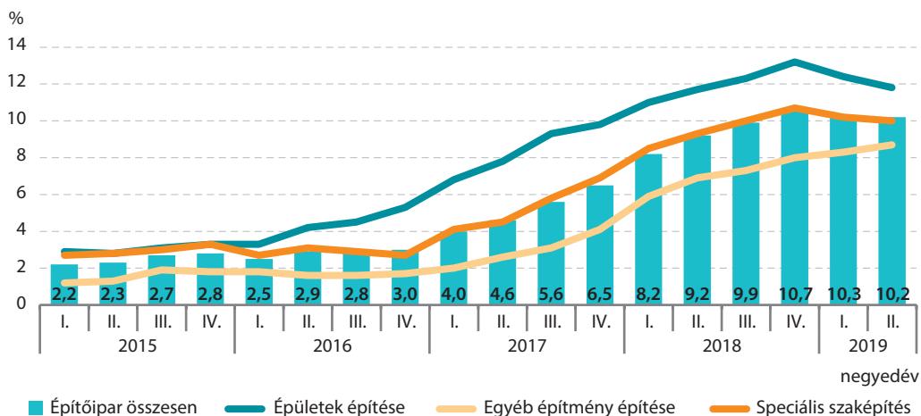
22. ábra Az építőipari árak változása ágazonként (az előző év azonos negyedévéhez képest)
