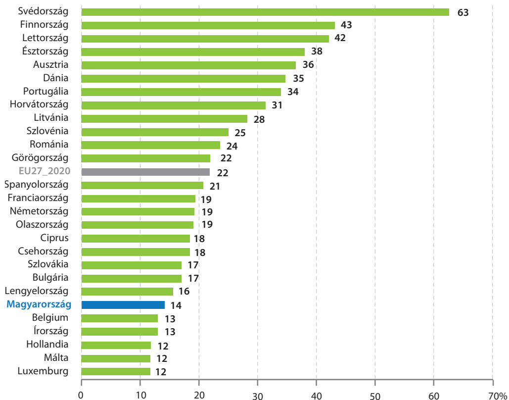
7.9. ábra A megújuló energiaforrások részesedése a teljes energiafelhasználásból az uniós tagországokban, 2021
