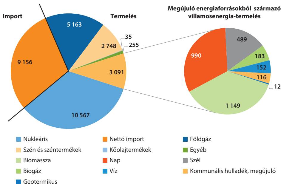
14. ábra Villamosenergia-felhasználás források szerint, 2019. január–augusztus, millió kWh
