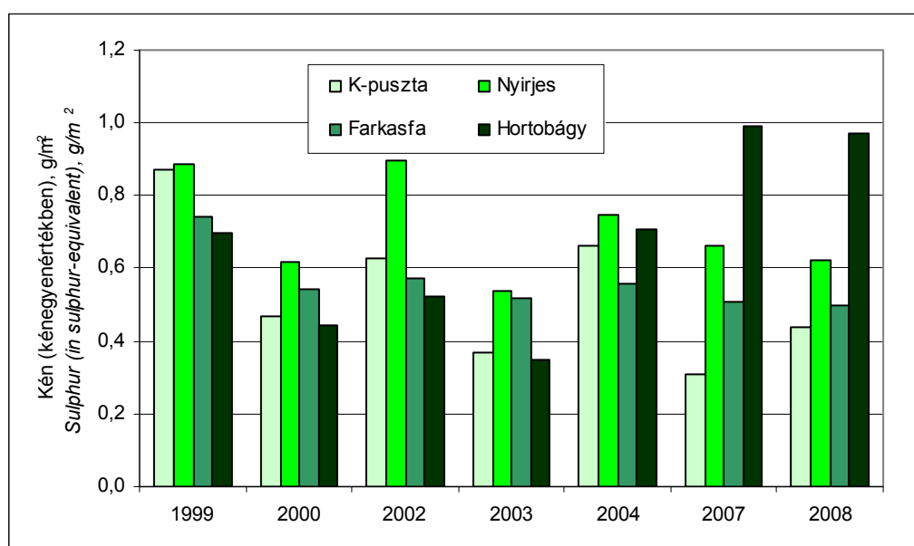
G 54 A kén nedves ülepedése Wet deposition of sulphur
