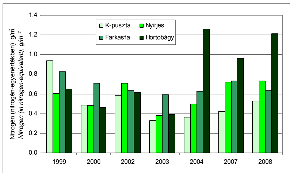
G 55 A nitrogén nedves ülepedése Wet deposition of nitrogen
