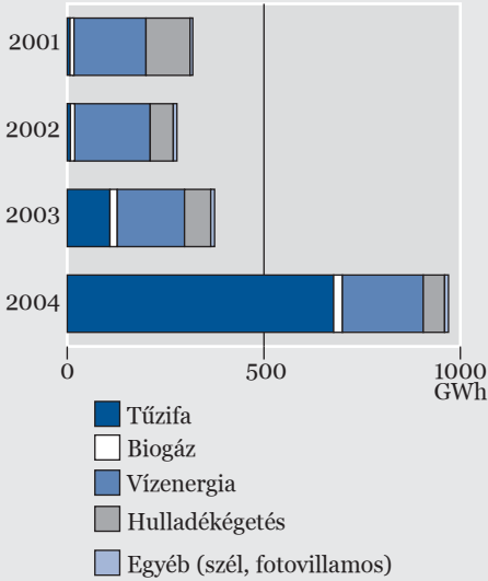
37. ábra Villamosenergia-termelés megújuló energiaforrásból Magyarországon
