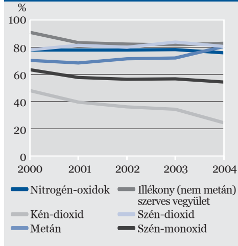
16. ábra Légszennyező anyagok kibocsátása Magyarországon (1990 = 100)
